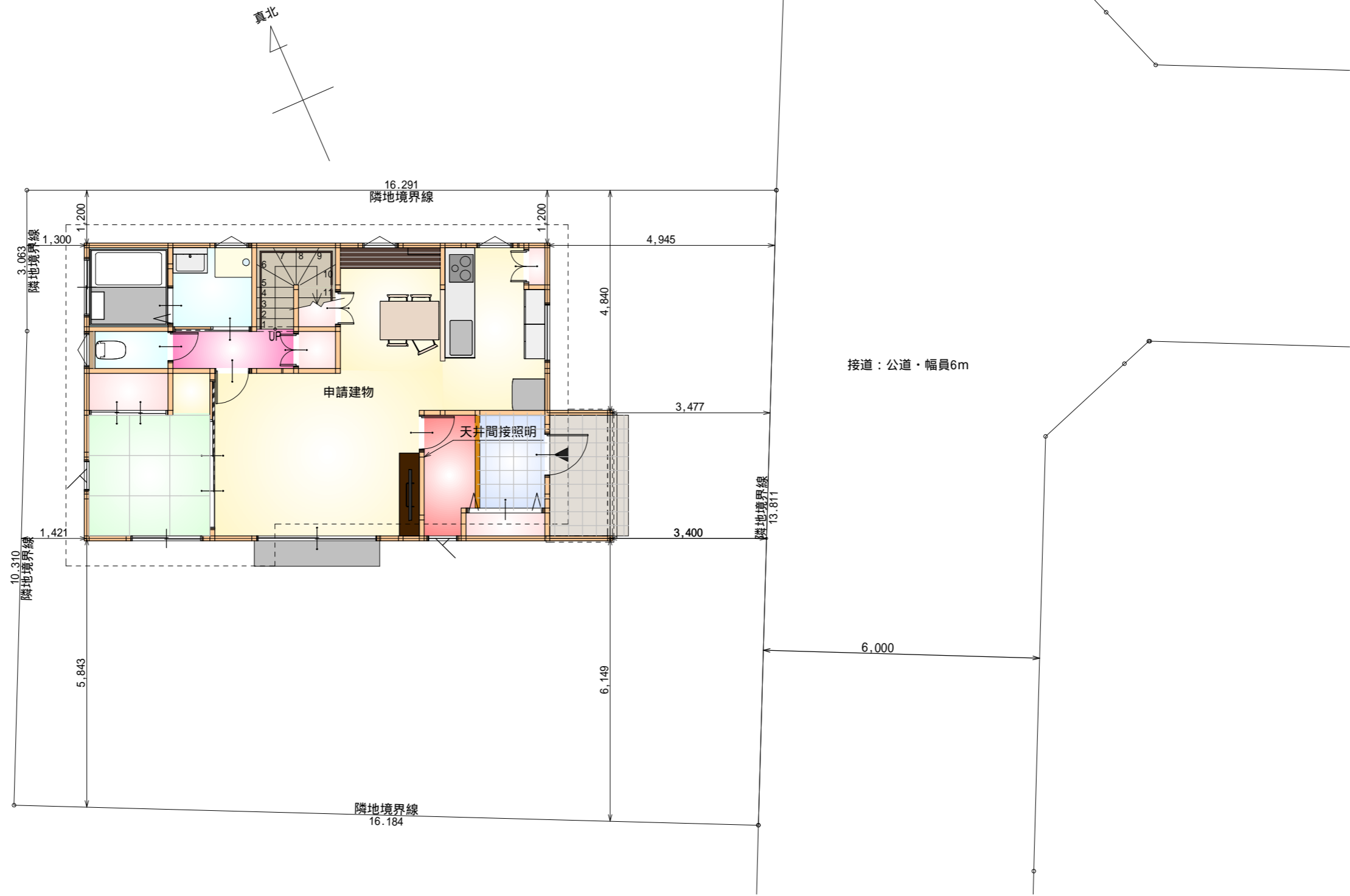
配置図 S:1/100
