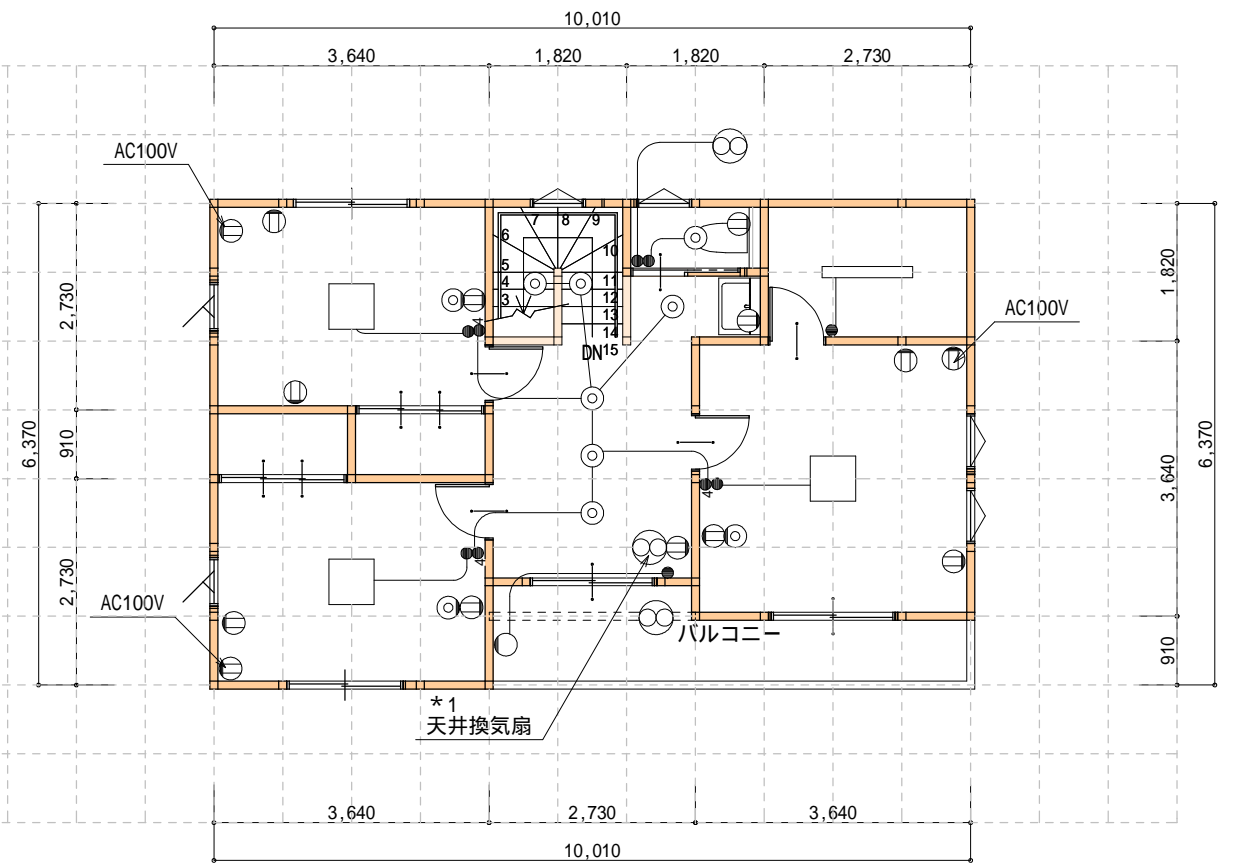
2階 電灯コンセント図 S:1/100
