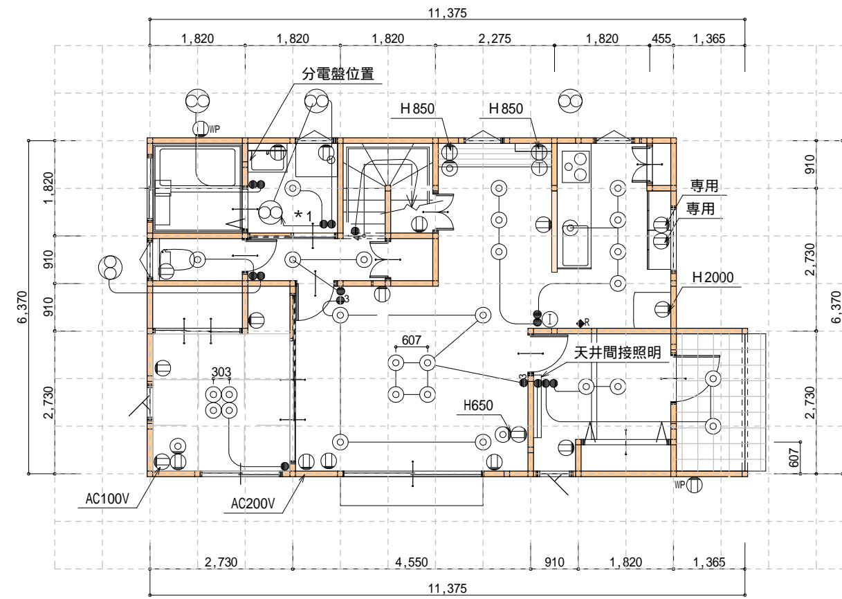
1階 電灯コンセント図 S:1/100
